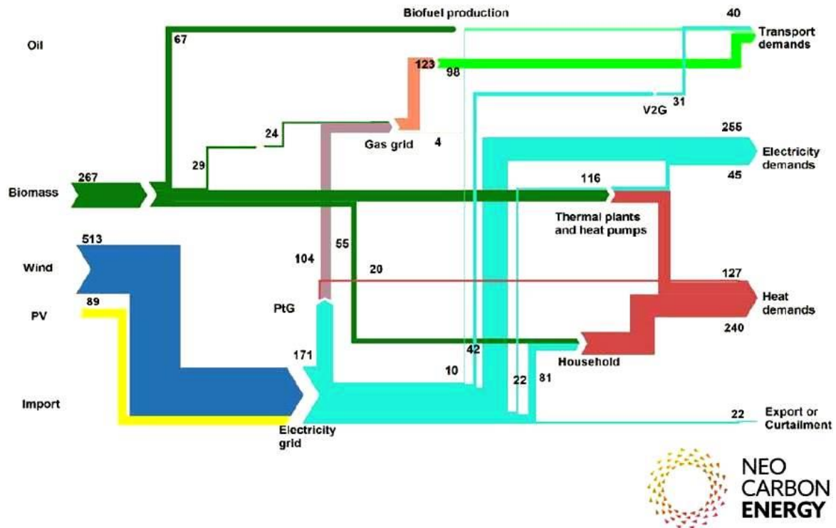
Figur 34. Scenario för framtida energiförsörjning för Åland baserad på 100 % förnyelsebar energi. (Källa: Child, M., Nordling, A., Breyer, C. Scenarios for a sustainable energy system in the Åland Islands in 2030. Energy Conversion and Management Vol. 137 (2017), 49-60.
